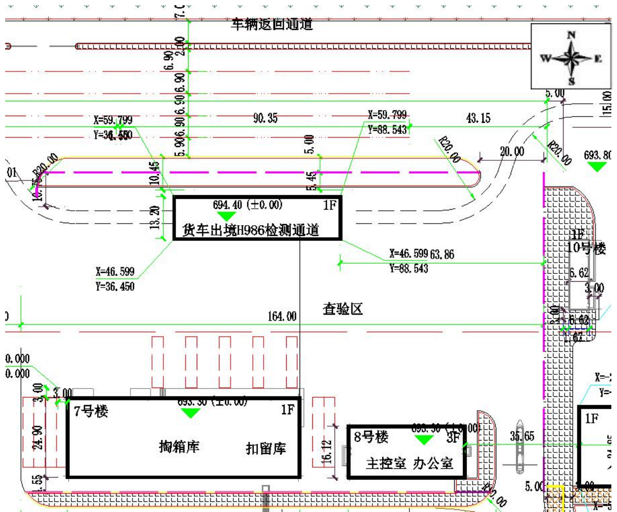
图 3 项目平面布局图
