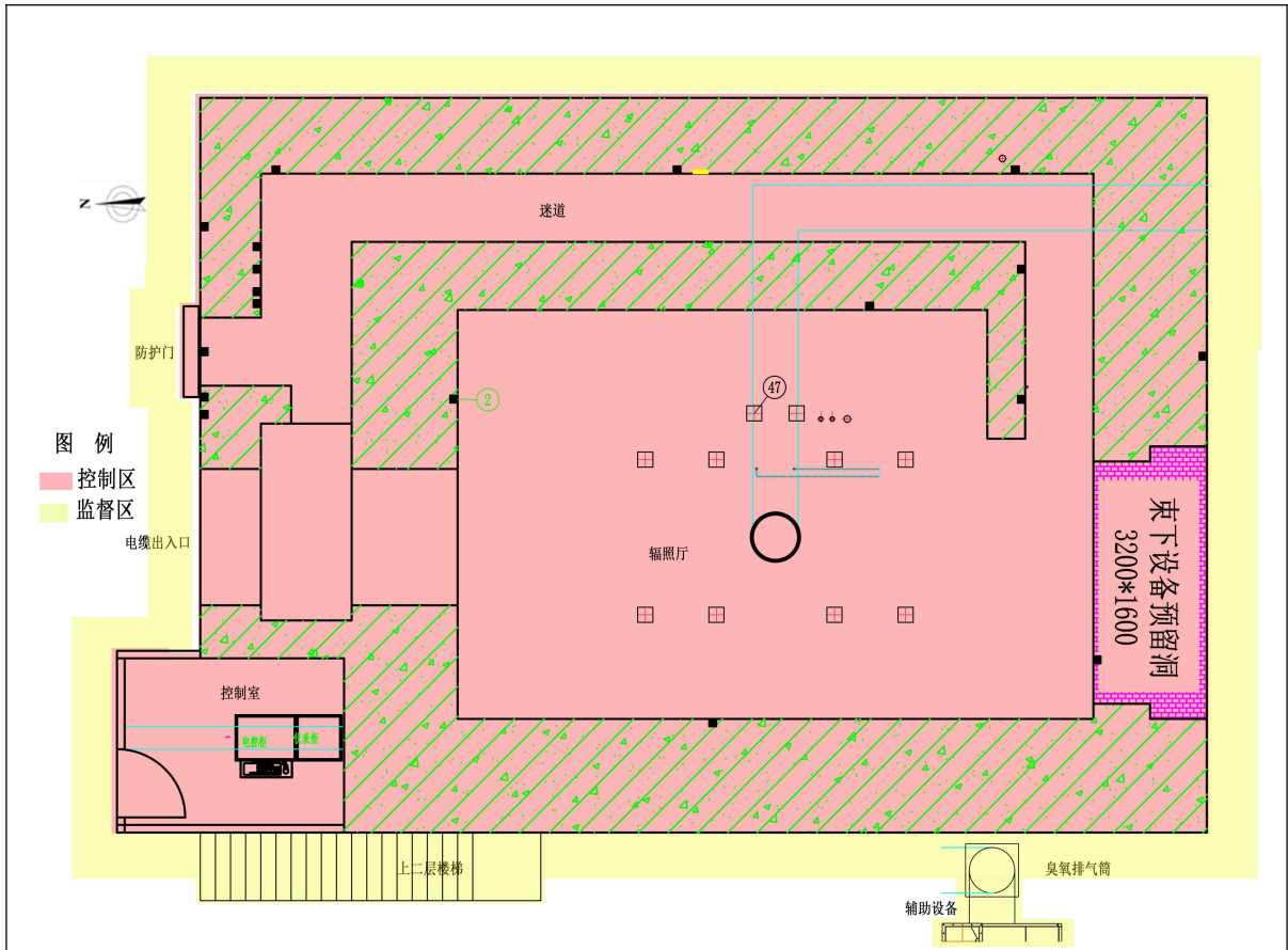
图10-2 辐照室一层辐照室平面布置及控制区和监督区划分示意图
