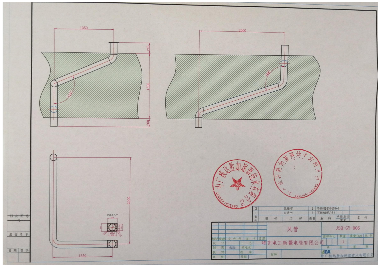
图 1-5 项目排风系统设计图
