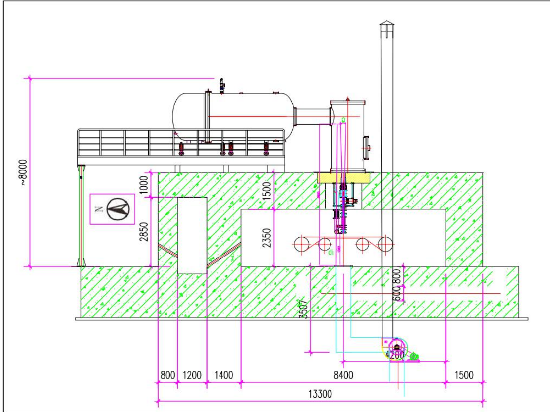
图10-5 本项目辐照室排风管道平面布设示意图
