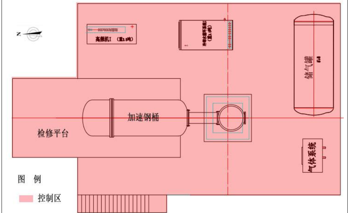
图10-3 辐照室一层辐照室平面布置及控制区和监督区划分示意图
