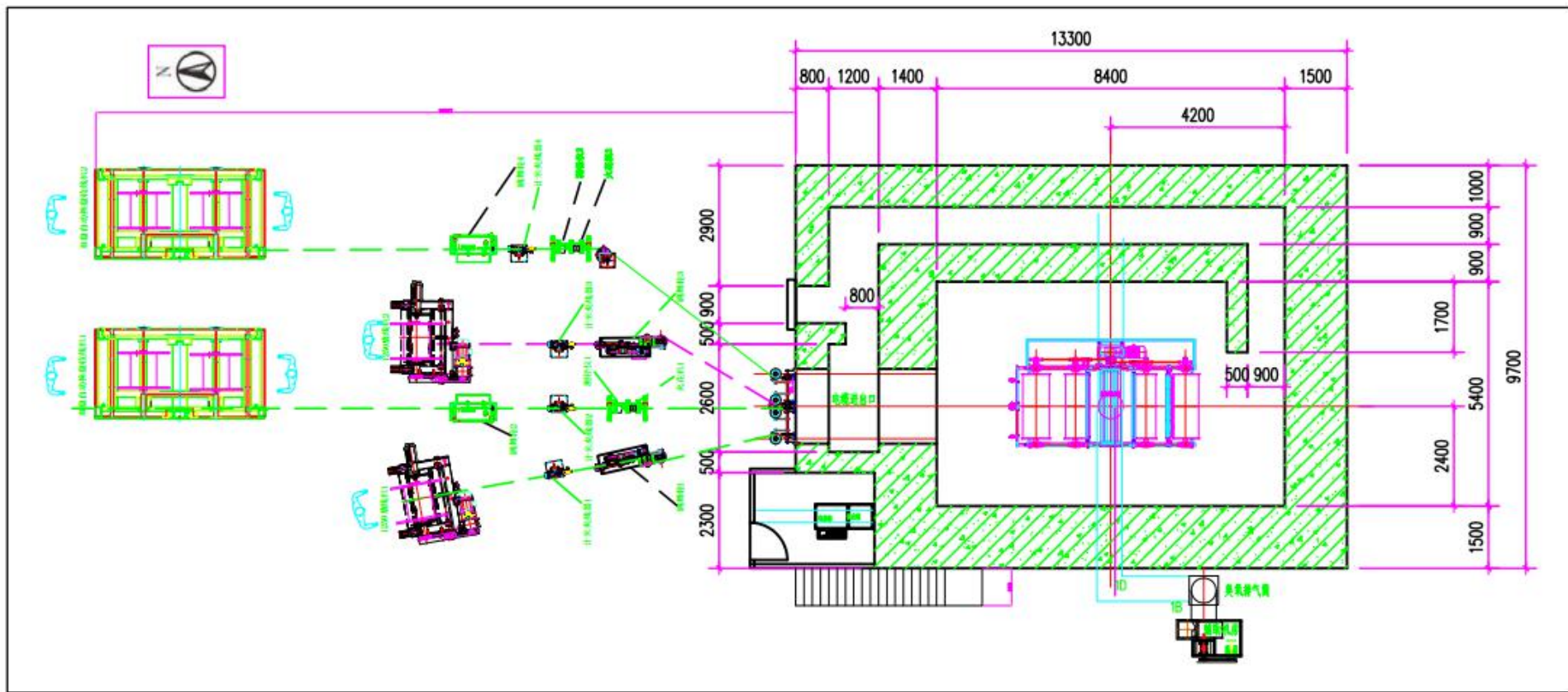
图 1-3 施工设计一层平面图
