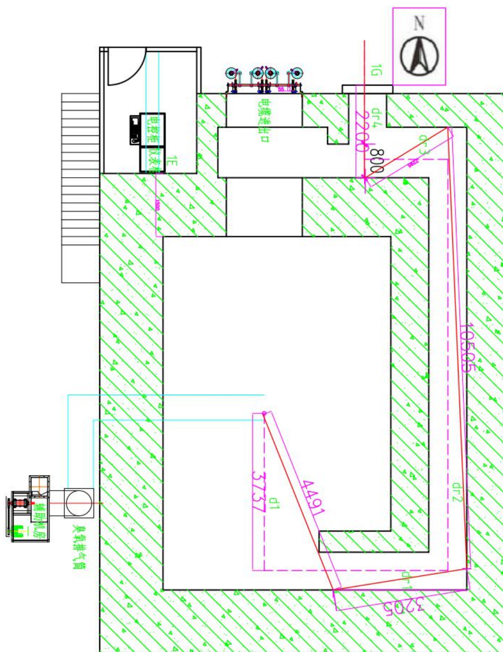
图11-2 辐照室散射路径示意图
