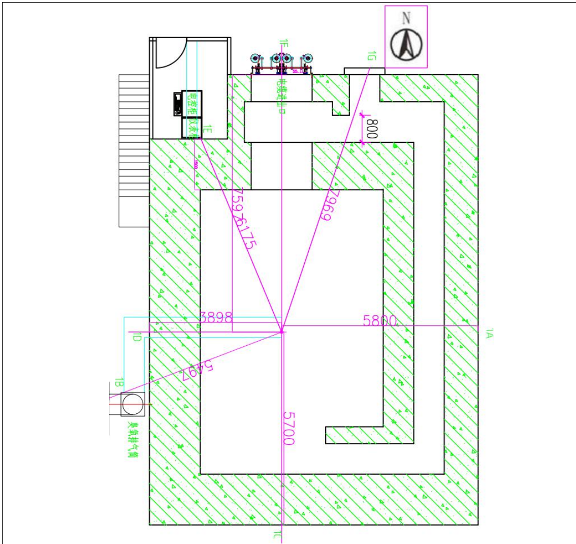
图 11-1 一层辐照室透射图
