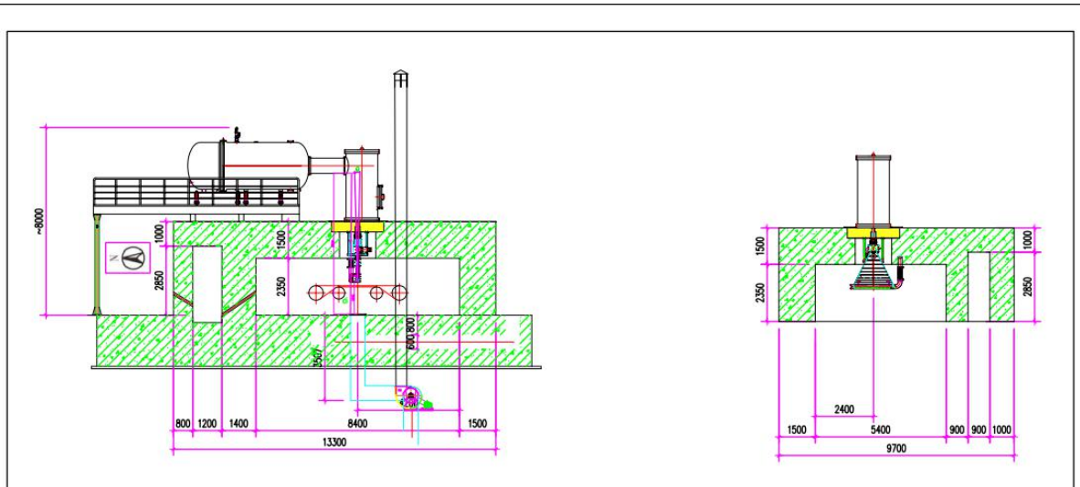
图10-4 本项目辐照室立面图
