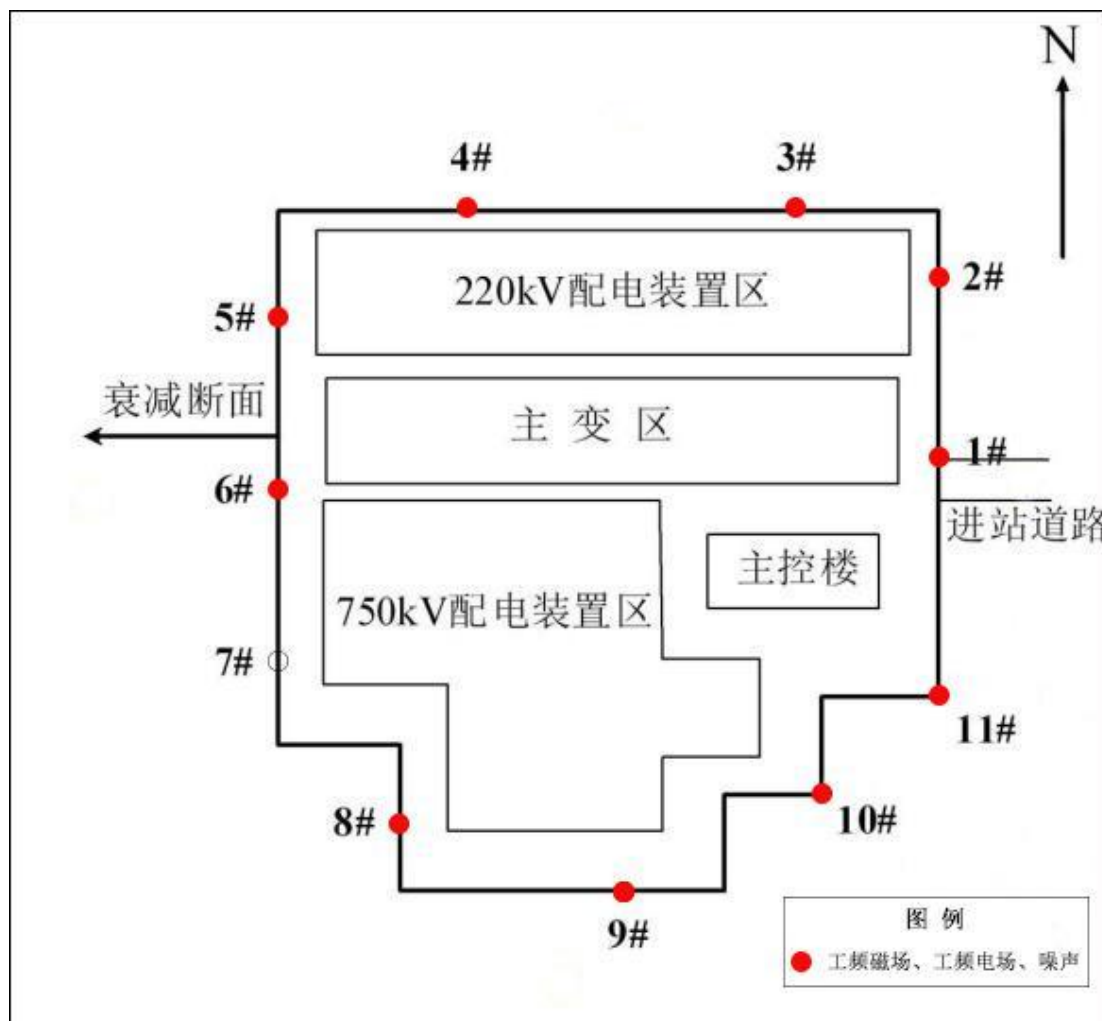
图 6.1-1 烟墩 750kV 变电站监测点位示意图
