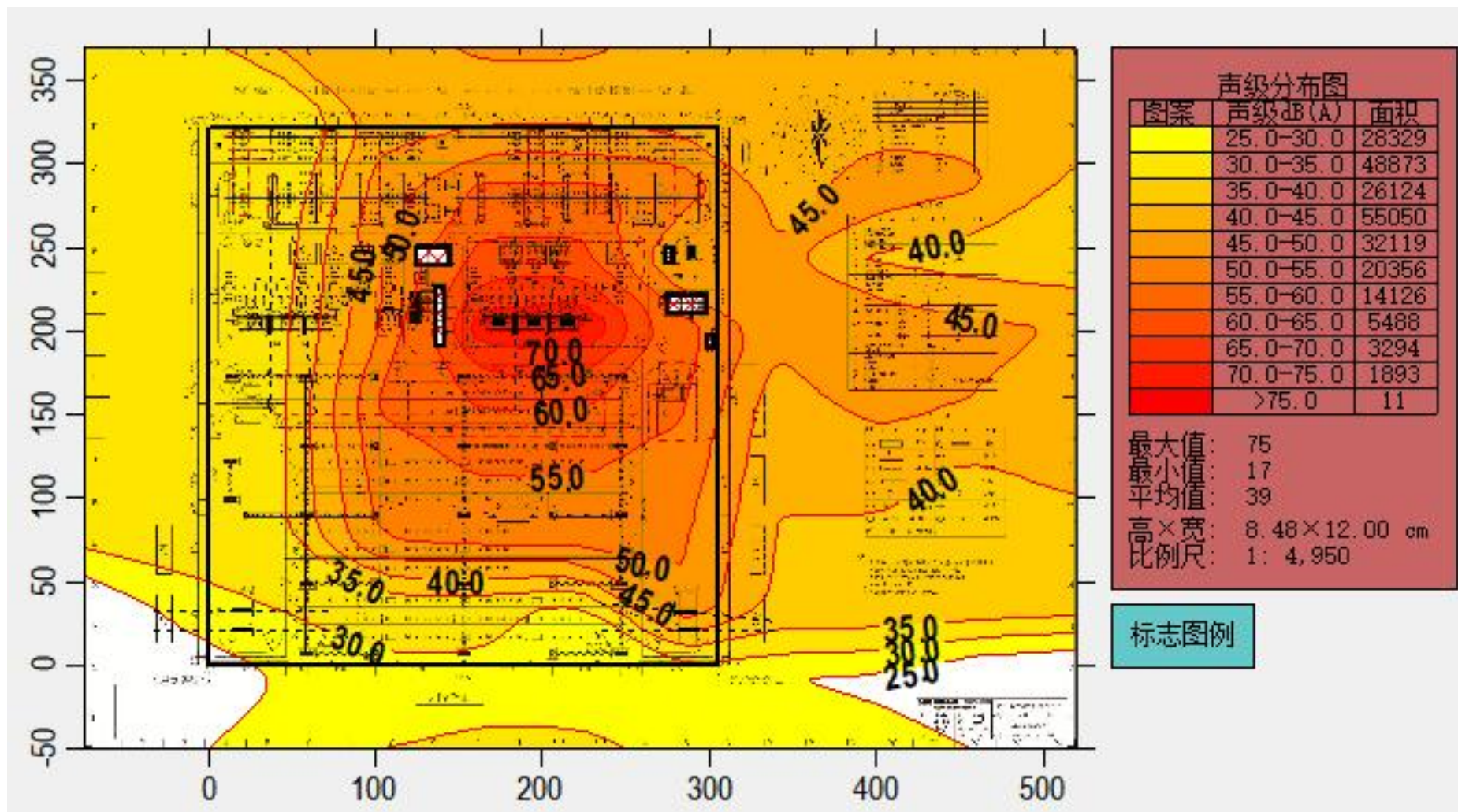
附图 9: 等声级线图
