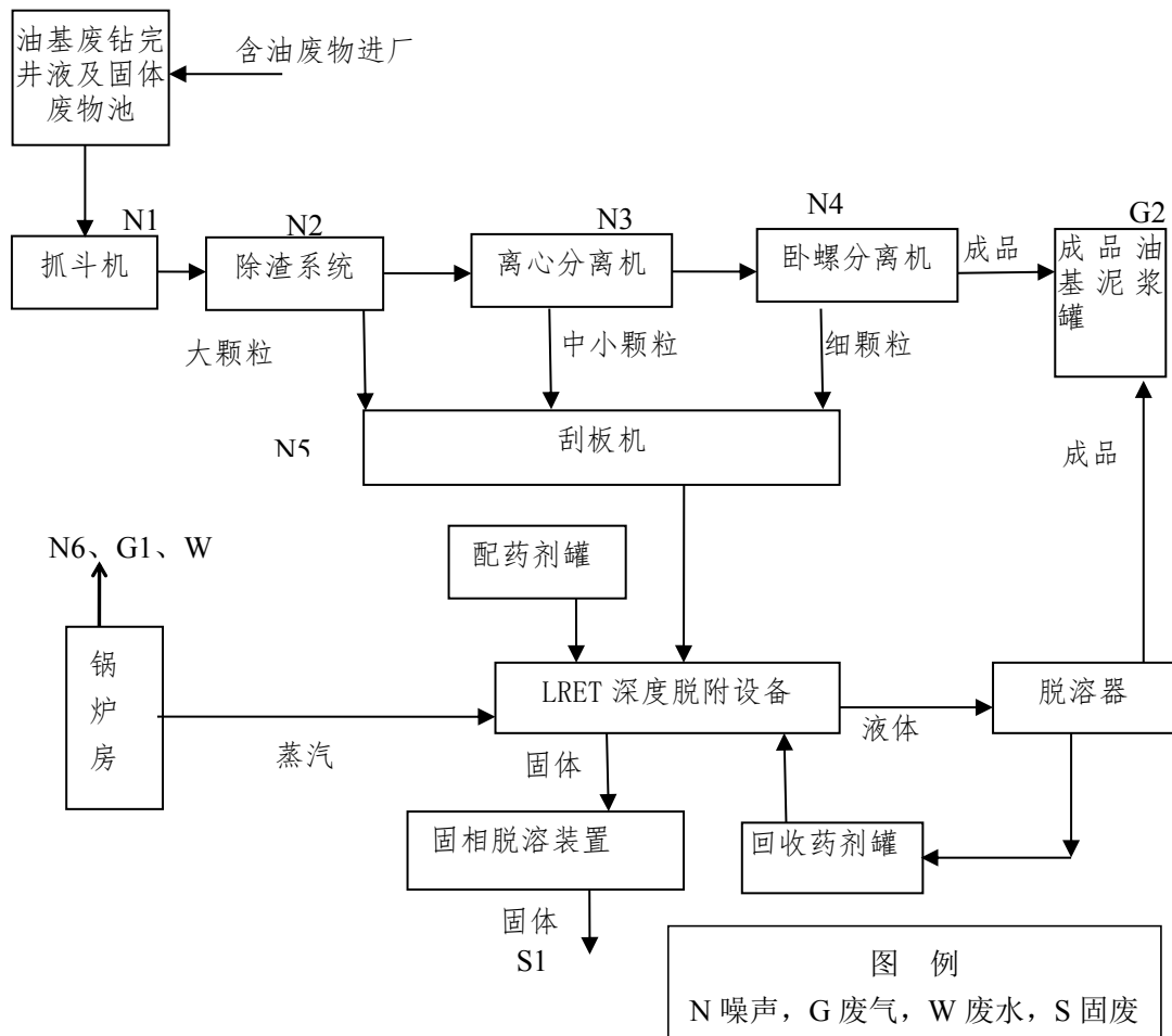
图 2.3-1 LRET 工艺生产流程图
