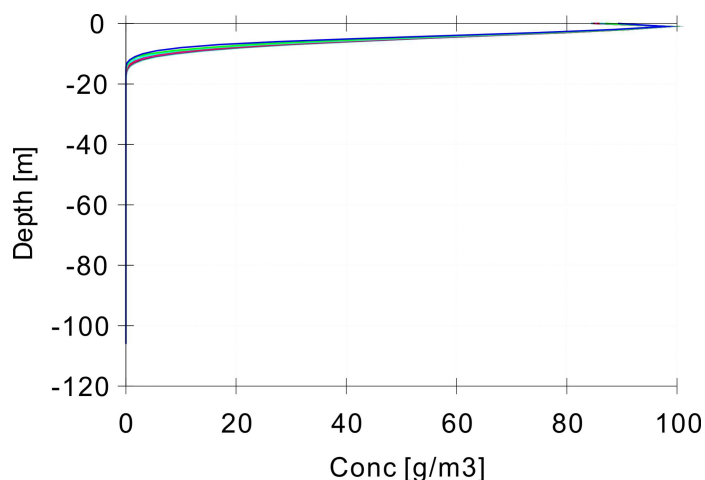
图 5.3-9 发生事故条件下各时间点石油类浓度随深度的变化
