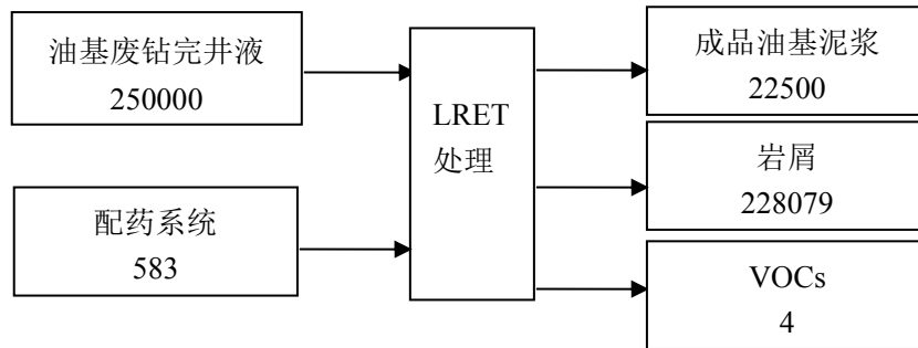
图 3.2-4 LRET 技术工艺流程图
