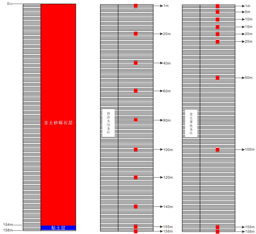
图 5.3-3 “含土砂砾石层—粘土层”模型分层、剖分和观测点位置
