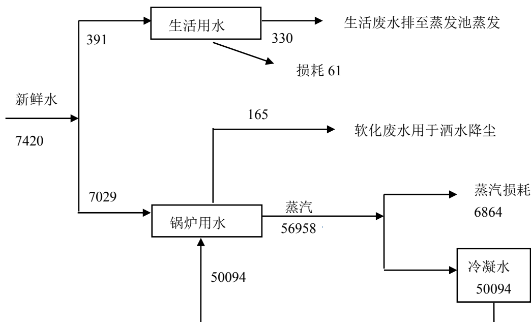
图 3.3-5 项目水衡图（单位：t/a）
