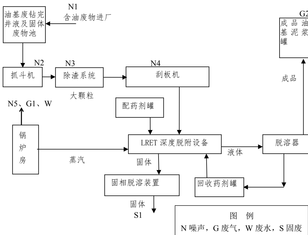
图 3.2-3 LRET 工艺生产流程图
