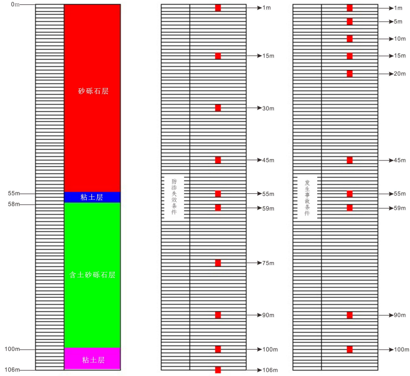
图 5.3-2 “砂砾石层—粘土层—含土砂砾石层—粘土层”模型分层、剖分和观测点位置
