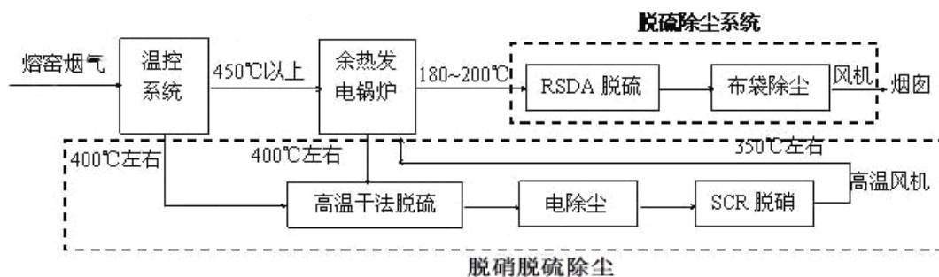
图 6.2-1 脱硫脱硝除尘系统工艺流程简图
