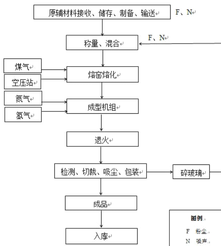
图 3.2-1 项目总工艺流程图
