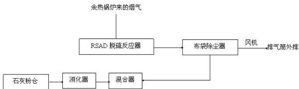
图 6.2-2 RSAD 脱硫与布袋除尘工艺流程示意图
