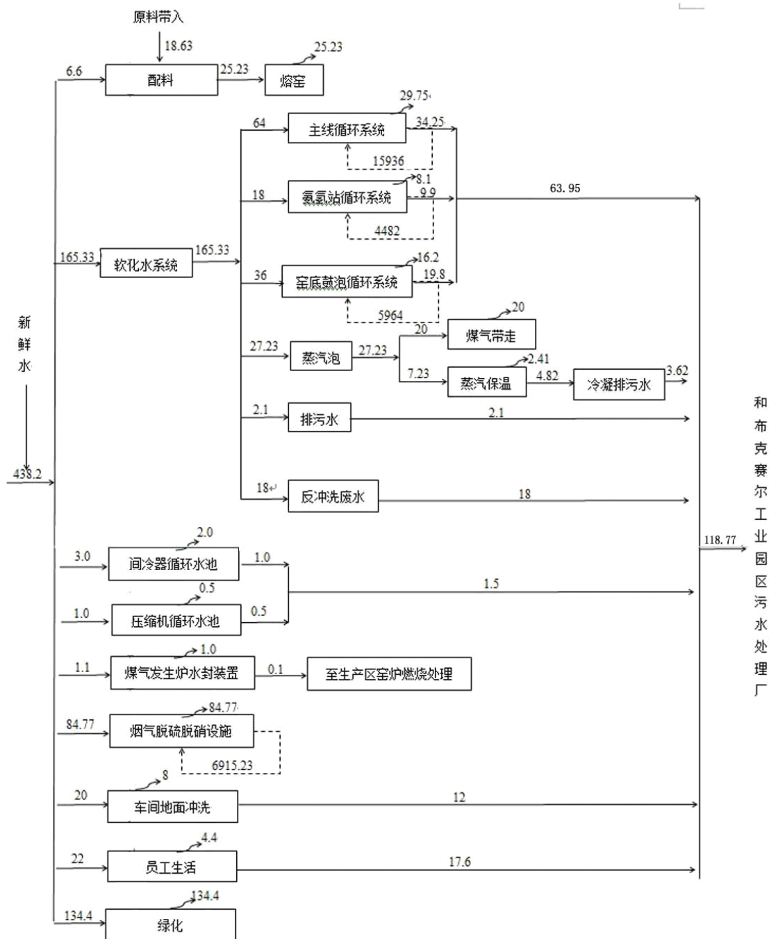
图 3.2-4 项目水平衡图 单位: m³/d
